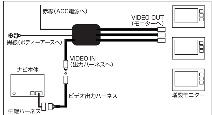
接続概要図
