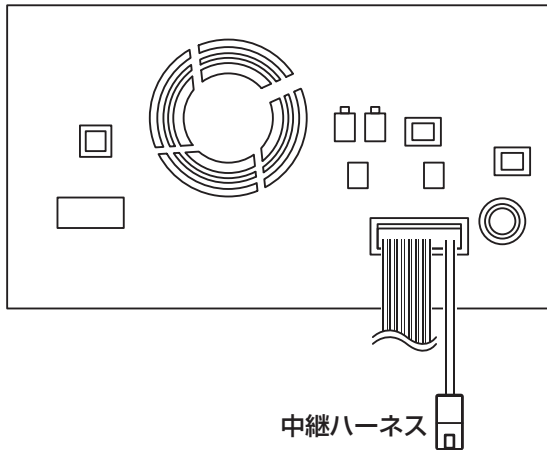
ナビ本体裏面図(イメージ)
