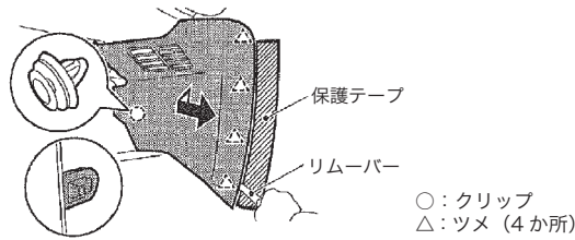
図2 助手席側ロアパネル取り外し
