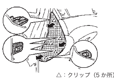
図8 助手席側サイドパネル取り外し
