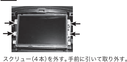
図14 モニターユニット取り外し、VHO-N40 接続位置
