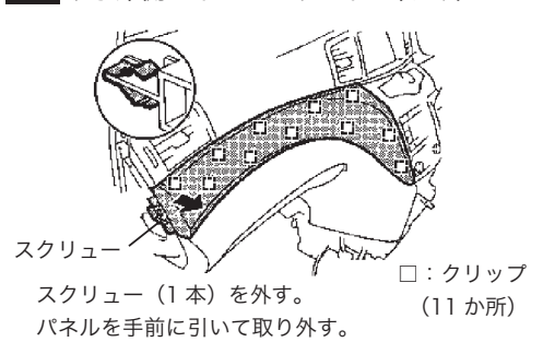
図9 助手席側フィニッシュパネル取り外し
