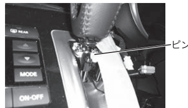
図11 シフトノブ取り外し
