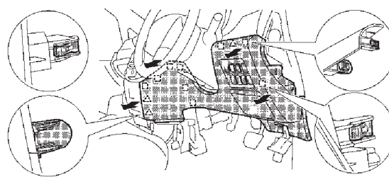
図6 ロアパネル取り外し
