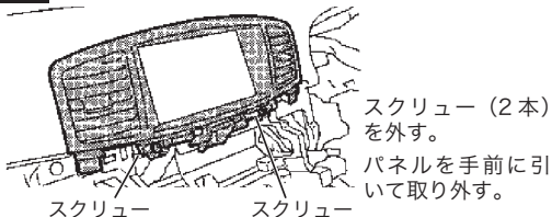
図13 クラスタパネル取り外し
