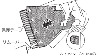
図1 運転席側ロアパネル取り外し
