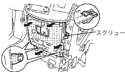
図7 インパネクラスター取り外し
