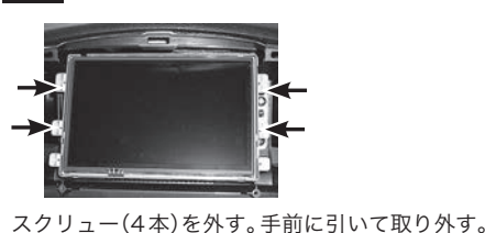
図14 モニターユニット取り外し、VHO-N40 接続位置
