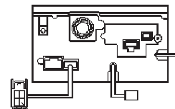
リアカメラハーネス接続位置 4ピンコネクタ （ナビ付属中継ハーネス）
