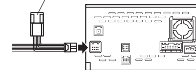
リアカメラハーネス接続位置 5ピンコネクタ
