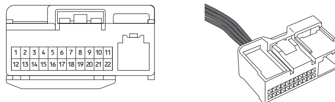
車両側カメラコネクタ(22ピンコネクタ)
