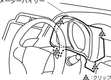
▲:クリップ
