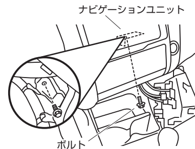
ボルト
