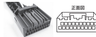
車両側カメラコネクタ(20ピンコネクタ)
