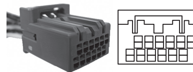
車両側カメラコネクタ(12ピンコネクタ)
