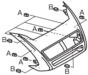
A:樹脂クリップ B:板金クリップ
